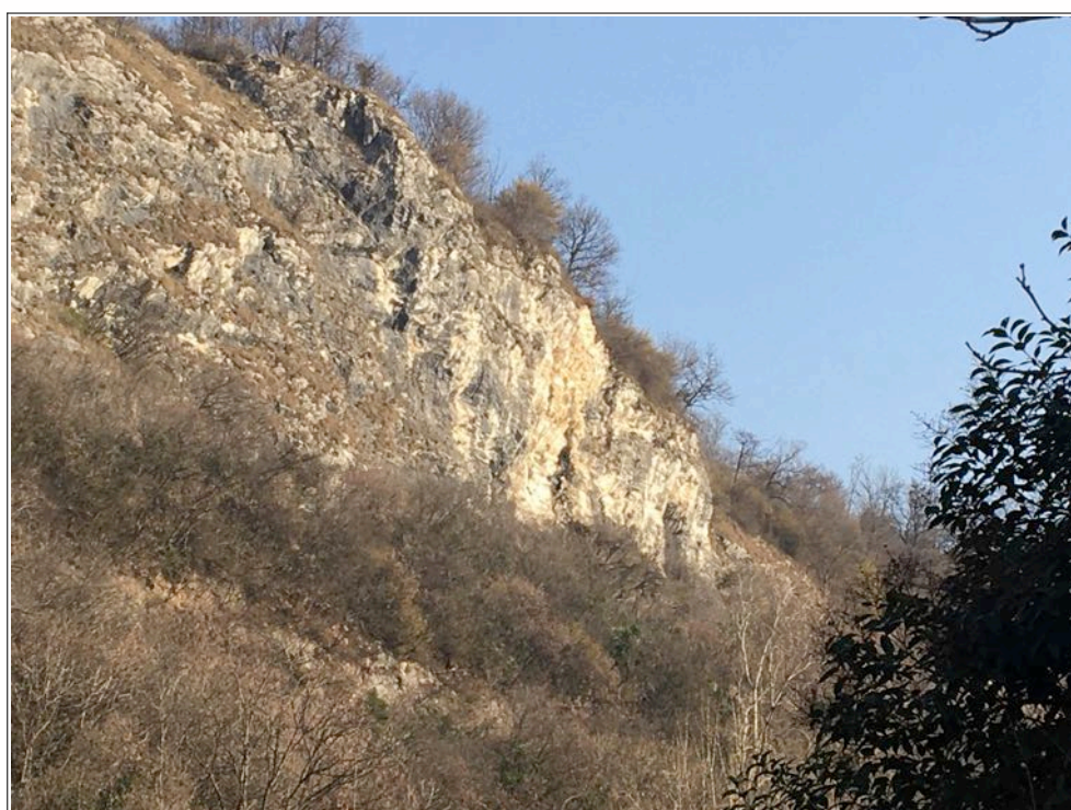
Figura 24 – Area da cui si sarebbero staccati i massi secondo la segnalazione pervenuta, vista dal piazzale della Chiesa Parrocchiale (foto del 05.03.2021).
